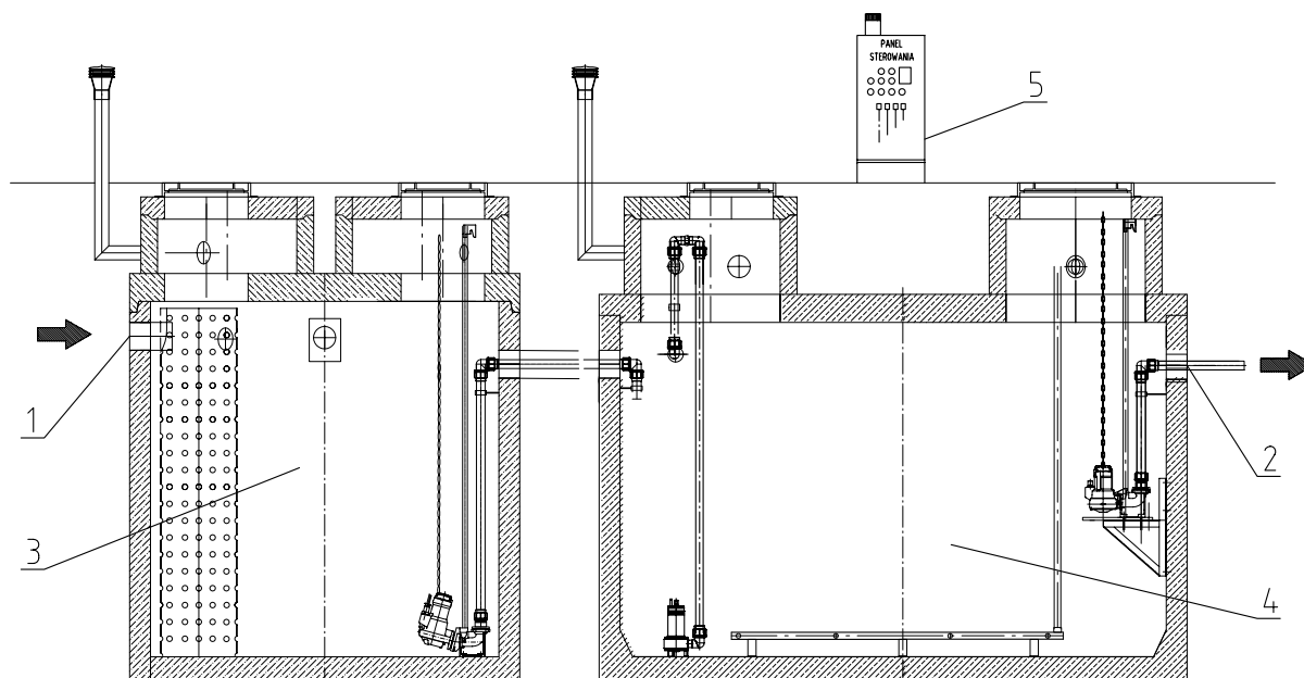
Oczyszczalnia ścieków NT-BIOS, rysunek poglądowy:
